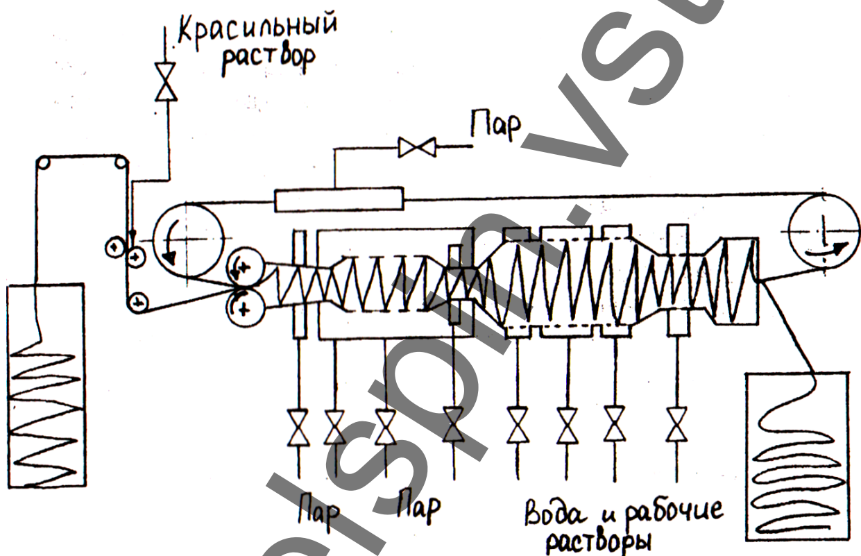
Рис. 4. Схема линии туннельного типа для непрерывного крашения волокна в жгуте
