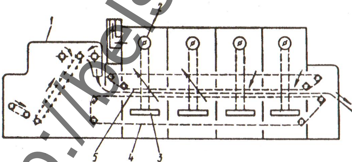
Рис. 5. Ленточная сушильная машина ЛС-1:
