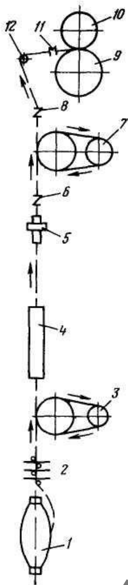
Рис. 12. Принципиальная схема однопроцессного способа получения высокоэластичимой нити
