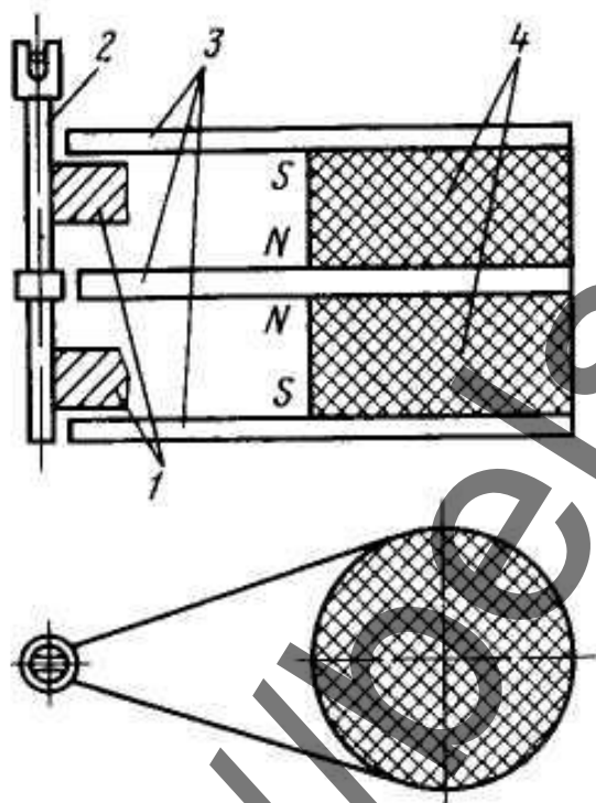
Рис. 17. Механизм ложного кручения, устанавливаемый на машинах ТК-500 и ТК-600
